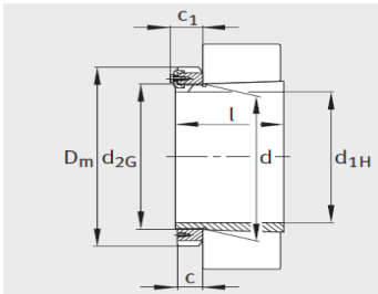
锥度为 1 : 12 (H240 系列, 锥度为 1 : 30) 止动卡板 MS30
