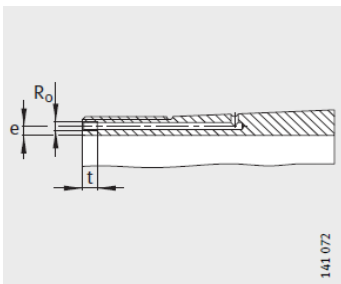
液压紧定套 (后缀 HG) 安装尺寸
